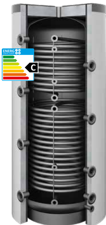
fol. 40 SG(B) 1000 z dwiema wężownicami w izolacji rozbieralnej
