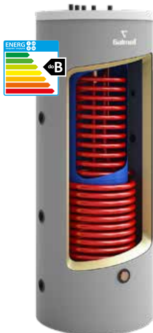
fol. 25 SG(K) Kumulo z dwiema wężownicami
