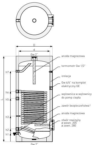
schemat wymiennika SGW(S) Maxi 700-1500
