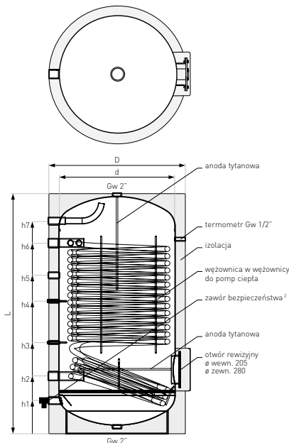
schemat wymiennika SGW(S) Maxi 800-1500
