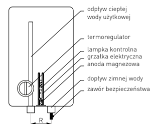
schemat ogrzewacza SG Fox 5-10 (nadumywalkowy)
