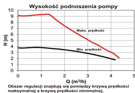
Dostępne zewnętrzne ciśnienie statyczne VS Natężenie przepływu
