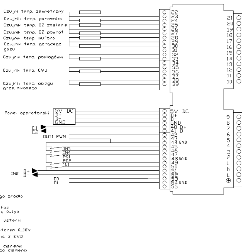
Rysunek 8 Złącza wejściowe/ panelu sterującego/ modułu internetowego/ czujników temperatur
