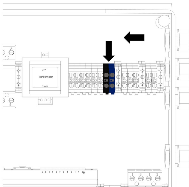
Rysunek 11 Miejsce podłączenia grzałki zbiornika (BH)
