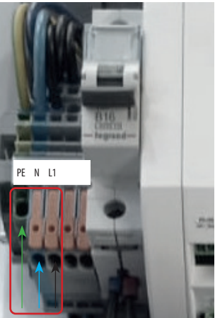
Rys. 90. Podłączenie zasilania Gbox 400 V (1 faza)
