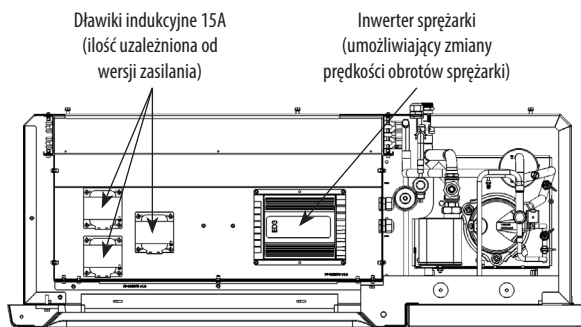
Rys. 18. Budowa wewnętrzna Airmax³ 12GT - widok z góry
