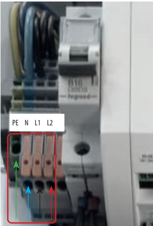
Rys. 89. Podłączenie zasilania Gbox 400 V (2 fazy)
