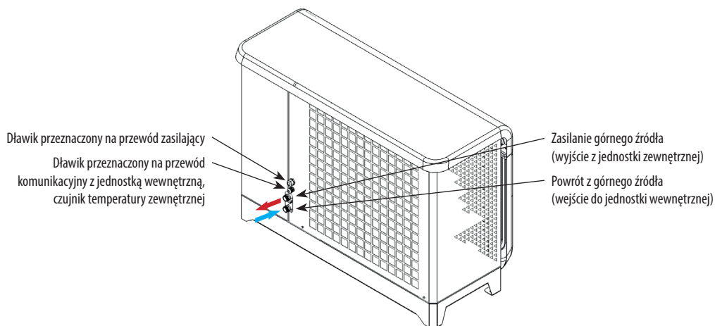
Rys. 9. Pompa ciepła Airmax³ - widok z tyłu
