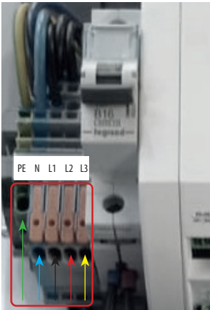
Rys. 88. Podłączenie zasilania Gbox 400 V (3 fazy)
