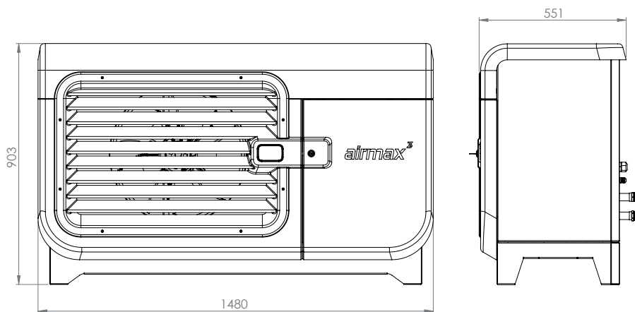
Rys. 10. Wymiary Airmax³ 7GT - widok z przodu i z boku
