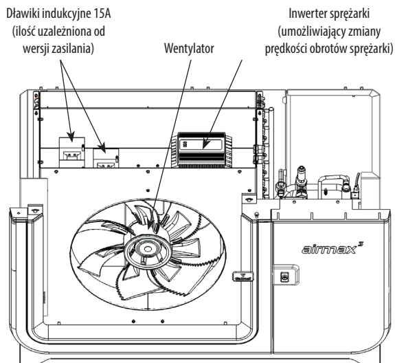
Rys. 17. Budowa wewnętrzna Airmax³ 12GT - widok od góry i przodu
