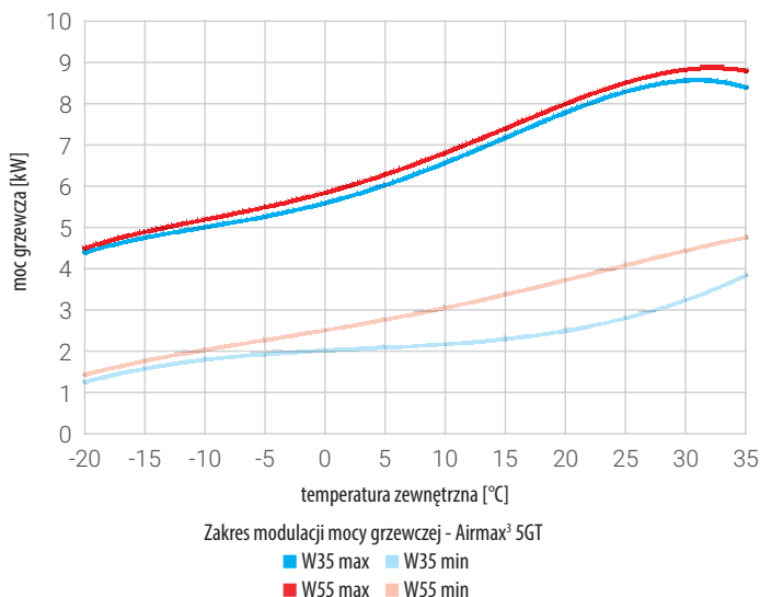
Wykres 2. Moc grzewcza (obroty minimalne i maksymalne sprężarki) dla zastosowań niskotemperaturowych (W35) i wysokotemperaturowych (W55) - pompa ciepła Airmax 3 SGT
