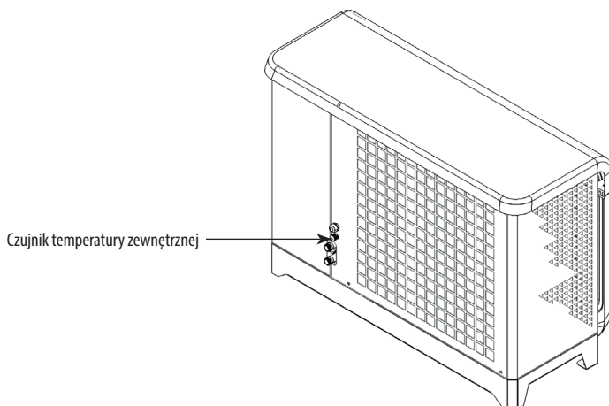
Rys. 5. Czujnik zewnętrzny pompy ciepła Airmax³
