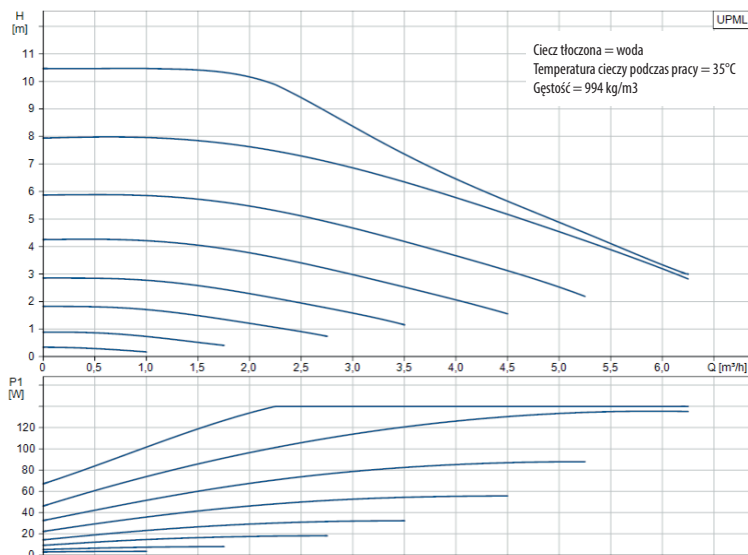
Wykres 14. Charakterystyki pompy obiegowej UPML GEO 25-105 130- czynniki: woda
