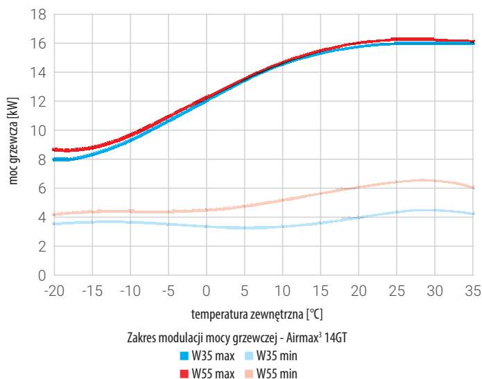
Wykres 11. Moc grzewcza (obroty minimalne i maksymalne sprężarki) dla zastosowań niskotemperaturowych (W35) i wysokotemperaturowych (W55) - pompa ciepła Airmax 3 14GT
