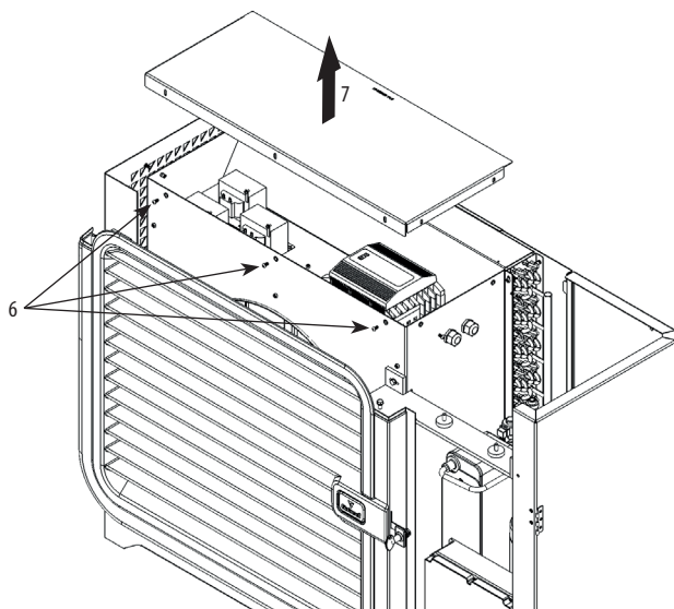
Rys. 59. Demontaż pokrywy komory inwertera Airmax 3
