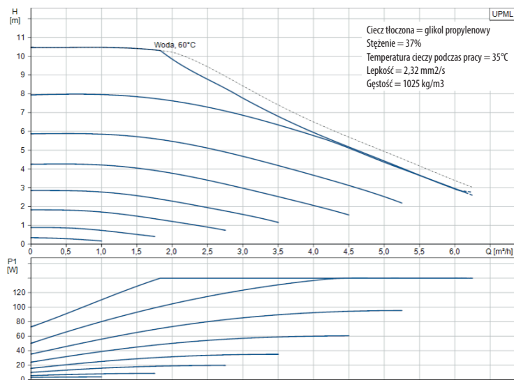
Wykres 15. Charakterystyki pompy obiegowej UPML GEO 25-105 130- czynniki: glikol propylenowy o stężeniu 37%, temperatura krzepnięcia -20°C
