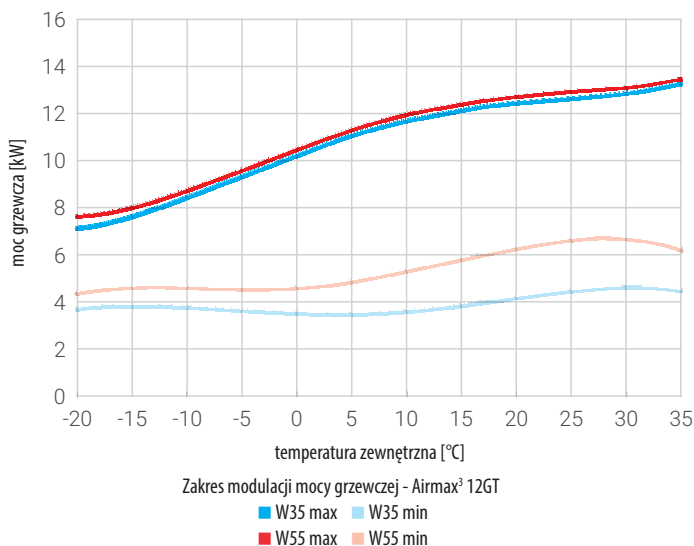
Wykres 8. Moc grzewcza (obroty minimalne i maksymalne sprężarki) dla zastosowań niskotemperaturowych (W35) i wysokotemperaturowych (W55) - pompa ciepła Airmax 3 12GT
