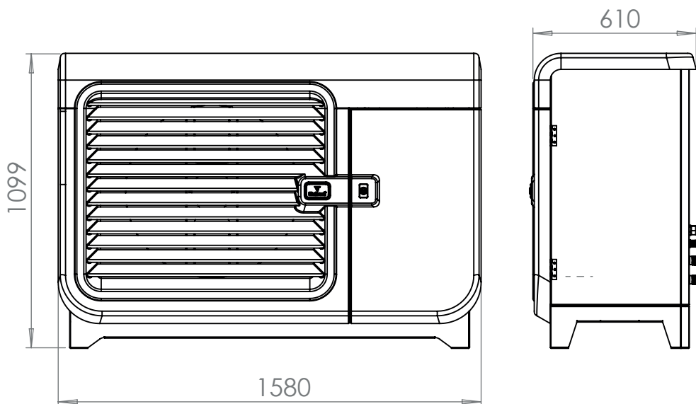
Rys. 12. Wymiary Airmax³ 12-14GT widok z przodu i z boku
