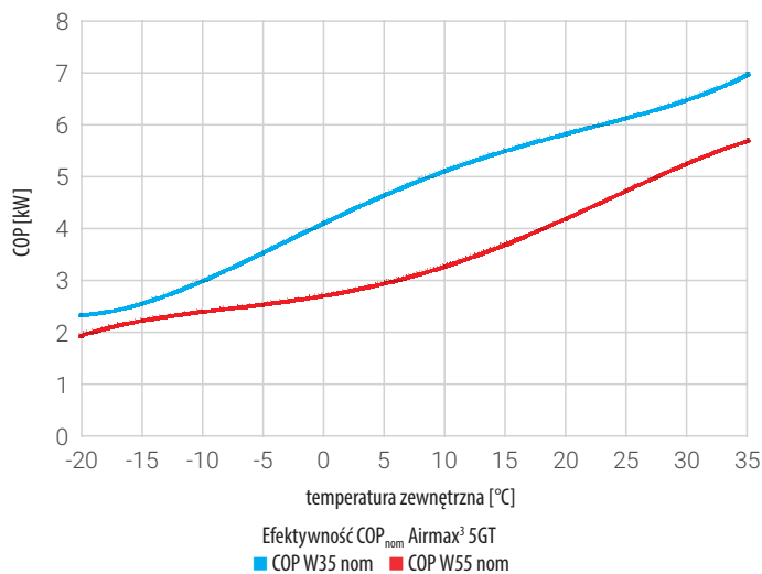
Wykres 4. COP (obroty nominalne sprężarki) dla zastosowań niskotemperaturowych (W35) i wysokotemperaturowych (W55) - pompa ciepła Airmax³ 5GT
