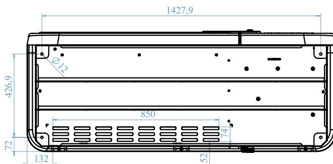
Rys. 37. Otwory montażowe Airmax³ 12-14GT - umiejscowienie na fundamencie
