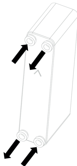
Rys. 73. Przeciwwąadowe podłączenie wymiennika płytowego
