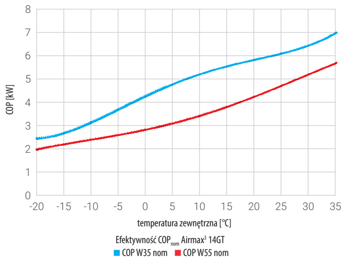
Wykres 13. COP (obroty nominalne sprężarki) dla zastosowań niskotemperaturowych (W35) i wysokotemperaturowych (W55) - pompa ciepła Airmax³ 14GT
