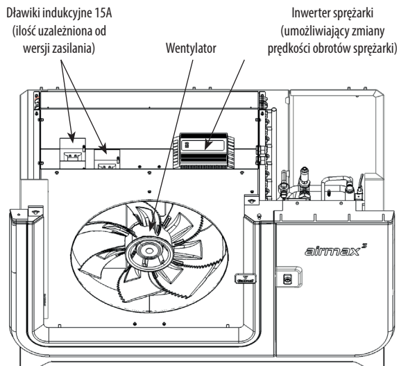
Rys. 17. Budowa wewnętrzna Airmax³ 12-14GT - widok od góry i przodu
