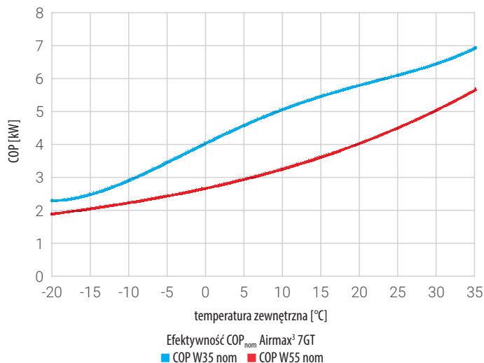
Wykres 7. COP (obroty nominalne sprężarki) dla zastosowań niskotemperaturowych (W35) i wysokotemperaturowych (W55) - pompa ciepła Airmax 3 7GT
