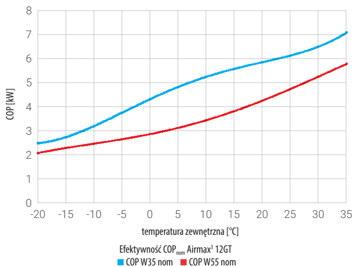
Wykres 10. COP (obroty nominalne sprężarki) dla zastosowań niskotemperaturowych (W35) i wysokotemperaturowych (W55) - pompa ciepła Airmax³ 12GT
