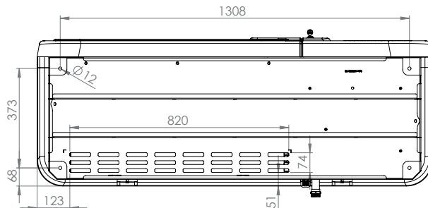
Rys. 36. Otwory montażowe Airmax³ 5-7GT - umiejscowienie na fundamencie
