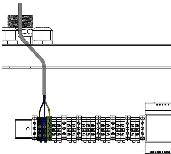
Rysunek 22 Miejsce podłączenia grzałki wspomagania (C.O) – grzałka bufora
