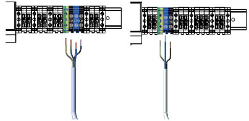
Rys. 16. Miejsce podłączenia siłownika mieszacza podłogówki SM4/5
