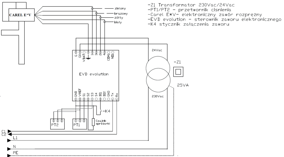
Rys. 13. Sterowanie zaworem rozprężnym
