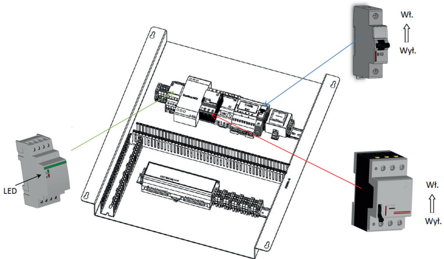
Rys. 20. Wyłącznik silnikowy sprężarki, bezpiecznik (pozycja wł./wytł.), czujnik kolejności i zaniku fazy (poprawne wskazanie diody LED- zielona)
