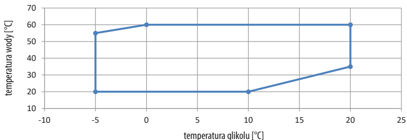
Wykres 1. Obszar pracy pompy ciepła Maxima Compact
