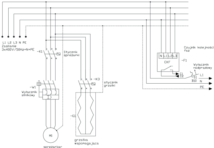
Rys. 11. Schemat zasilania głównego
