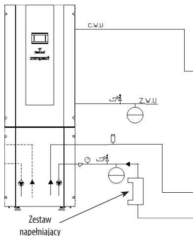
Rys. 5. Obieg grzewczy - górnego źródła
