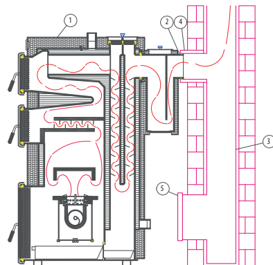
Rys. 8 - Podłączenie kotła do komina
