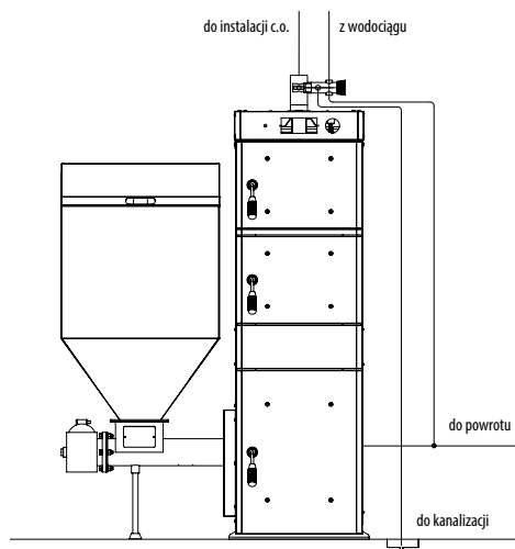
Rys. 7 - Kocioł Galaxia KWE z zaworem upustowo-schładzającym
