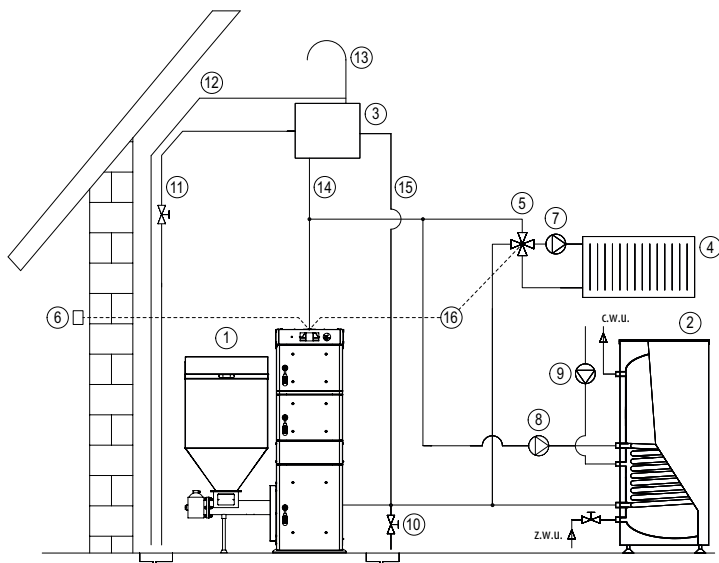
Rys. 5 - Poglądowy schemat podłączenia kotła Galaxia KWE do instalacji c.o.
