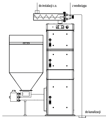
Rys. 6 - Kocioł Galaxia KWE z węzłownicą schładzającą
