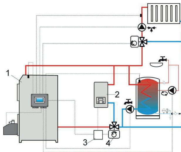
Rys. 18 5 Schemat hydrauliczny z kotłem rezerwowym w obiegu zamkniętym, gdzie: 1 – regulator, 2 – kocioł rezerwowy, 3 – przekaźnik (Rys. 20), 4 – zawór przełączający (z wyłącznikami krańcowymi).
