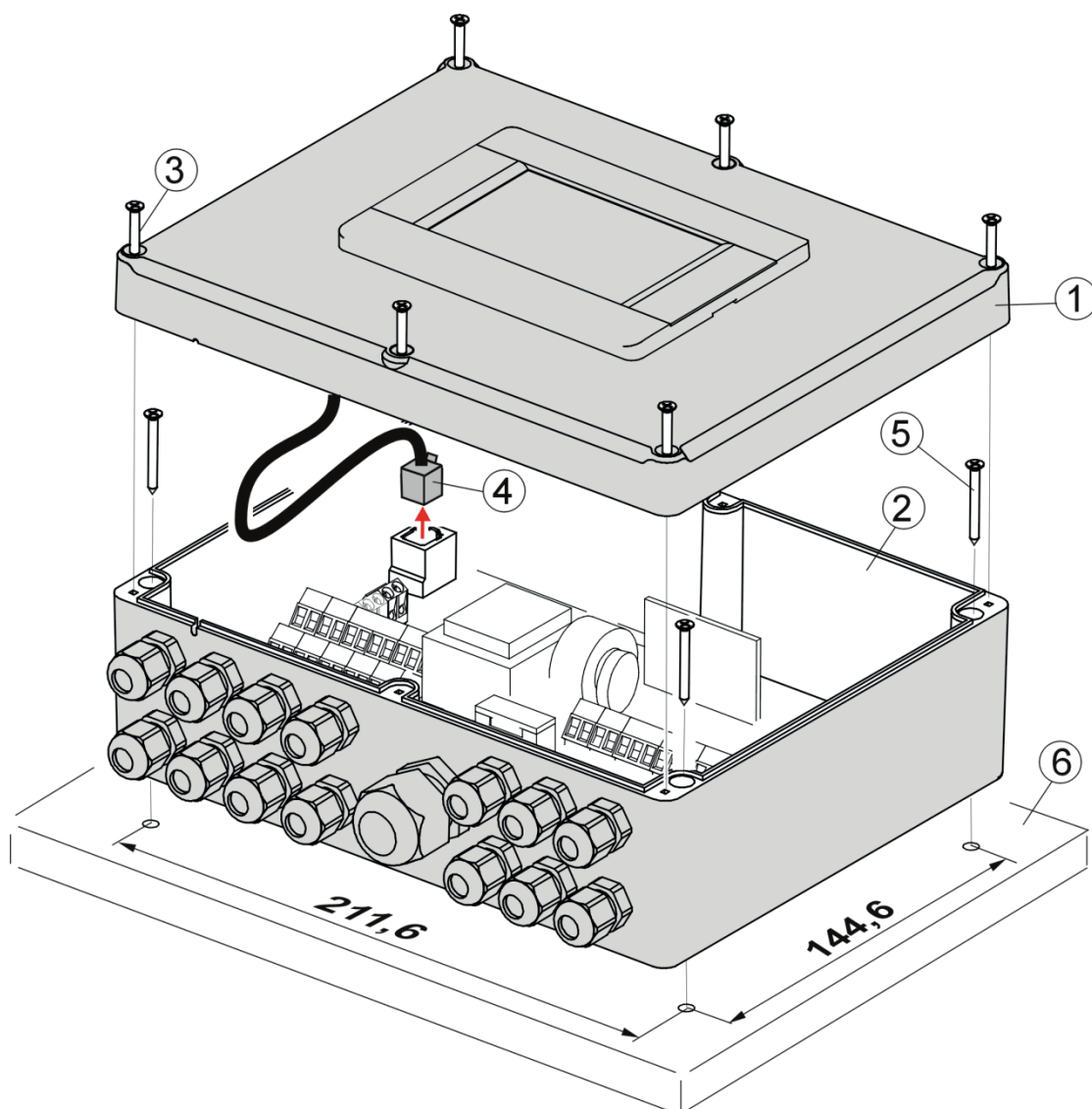
Rys. 13 Osadzenie regulatora na powierzchni montażowej, gdzie: 1 – pokrywa, 2 – podstawa, 3 – wkręt pokrywy, 4 – wtyk, 5 – wkręt mocujący do powierzchni montażowej, 6 – powierzchnia montażowa.
