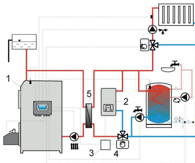
Rys. 19 6 Schemat hydrauliczny z kotłem rezerwowym w obiegu otwarto-zamkniętym, gdzie: 1 – regulator, 2 – kocioł rezerwowy, 3 – przekaźnik (Rys. 20), 4 – zawór przełączający (z wyłącznikami krańcowymi), 5 – wymiennik ciepła, zalecane ustawienie: priorytet CWU = wyłączony , wymiennik ciepła = TAK .
