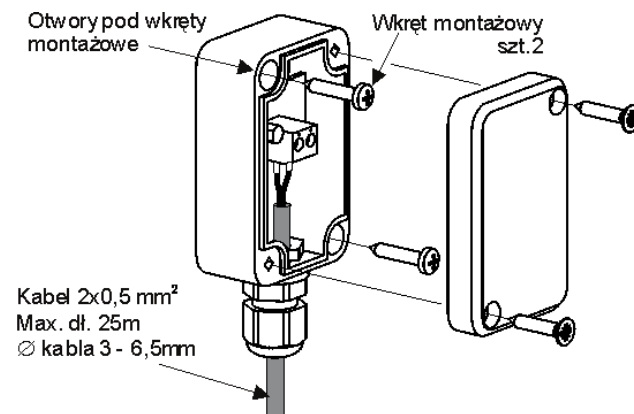
Rys. 16 Podłączenie czujnika pogodowego CT4-P.
