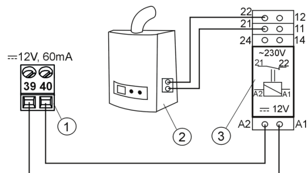
Rys. 17 Przykładowy schemat układu do podłączenia kotła rezerwowego do regulatora, gdzie: 1- moduł B, 2 – kocioł rezerwowo (gazowy lub olejowy), 3 –przekaźnik RM 84-2012-35-1012 i podstawka GZT80 RELPOL.
