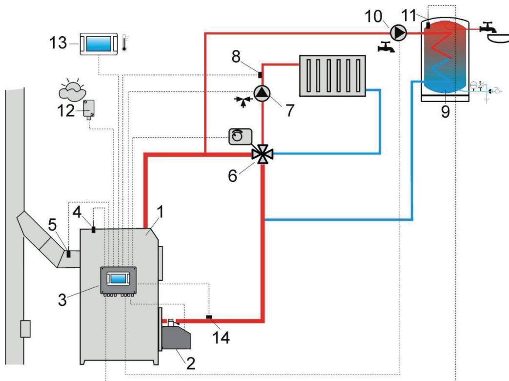
Rys. 10 Schemat z zaworem czterodrogowym sterującym obiegiem centralnego ogrzewania 1 , gdzie: 1 – kocioł, 2 – palnik, 3 – regulator, 4 – czujnik temperatury kotła CT4, 5 – czujnik temperatury spalin CT2S (tylko podgląd temperatury), 6 – siłownik zaworu czterodrogowego, 7 – pompa obiegu mieszacza, 8 – czujnik temperatury obiegu mieszacza, 9 – zasobnik ciepłej wody użytkowej, 10 – pompa ciepłej wody użytkowej, 11 – czujnik ciepłej wody użytkowej, 12 – czujnik temperatury pogodowy CT4-P, 13 – panel pokojowy ecoSTER-TOUCH lub standardowy termostat pokojowy, 14 – czujnik temperatury powrotu (nie jest niezbędny do działania układu).
