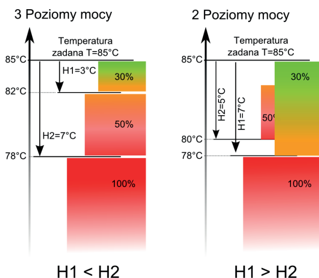
Rys. 4 Histerezy H1 i H2 modulacji mocy
