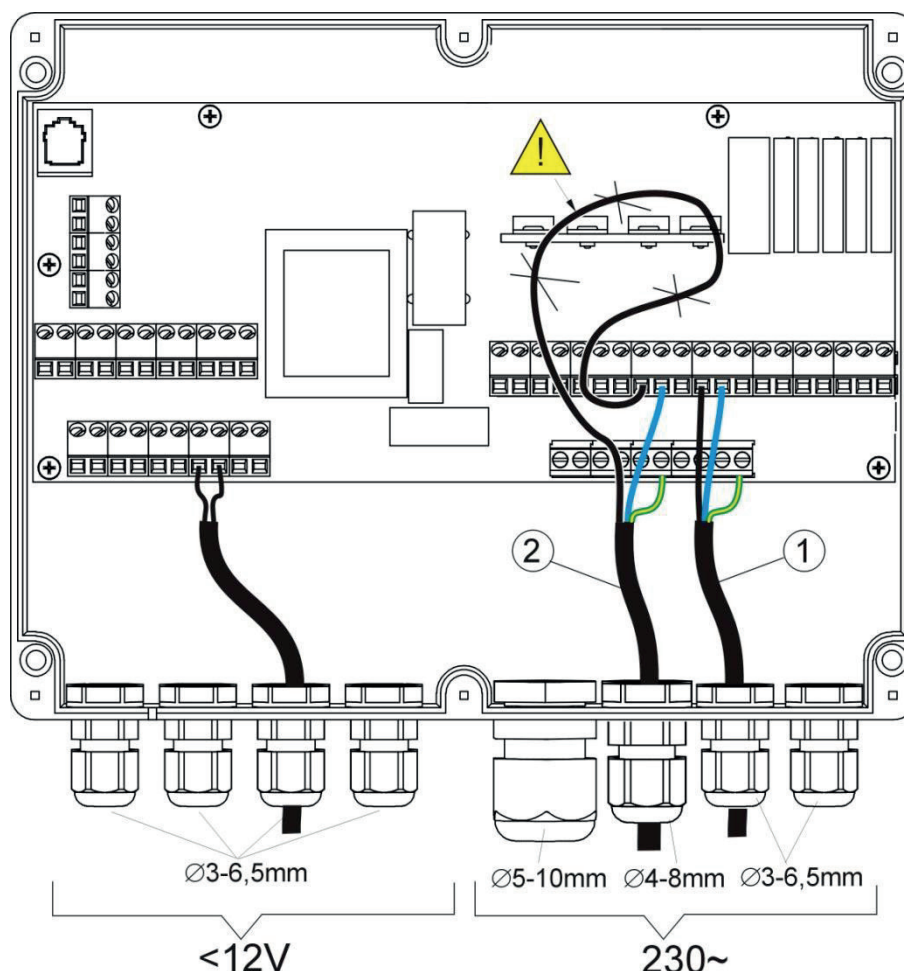
Rys. 14 Podłączanie przewodów, gdzie 1 – przewód podłączony poprawnie, 2 - przewód podłączony błędnie (nie dopuszcza się zwijania nadmiaru przewodów wewnątrz urządzenia).
