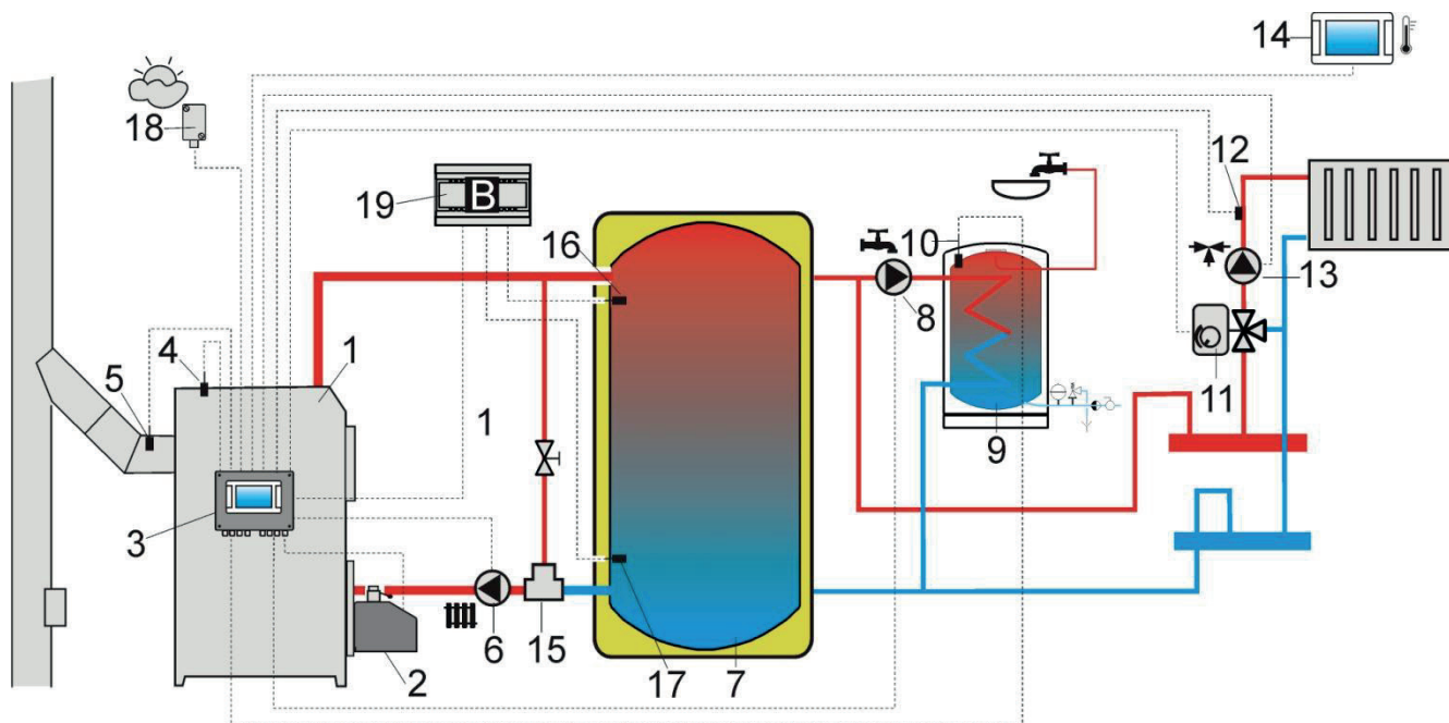
Rys. 11 Schemat z buforem cieplnym 2 , gdzie: 1 – kocioł, 2 – palnik, 3 – regulator, 4 – czujnik temperatury kotła, 5 – czujnik temperatury spalin (tylko podgląd temperatury), 6- pompa kotła, 7 – bufor ciepły, 8 – pompa ciepłej wody użytkowej, 9 - zasobnik ciepłej wody użytkowej, 10 – czujnik temperatury ciepłej wody użytkowej, 11 – siłownik zaworu mieszającego, 12 – czujnik temperatury obiegu mieszacza, 13 – pompa mieszacza, 14 – panel pokojowy ecoSTER-TOUCH z funkcją termostatu pokojowego, 15 – termostatyczny zawór trójdrogowy do ochrony powrotu, 16 – czujnik temperatury bufora górny, 17 – czujnik temperatury bufora dolny, 18 – pogodowy czujnik temperatury, 19 – dodatkowy moduł B.
