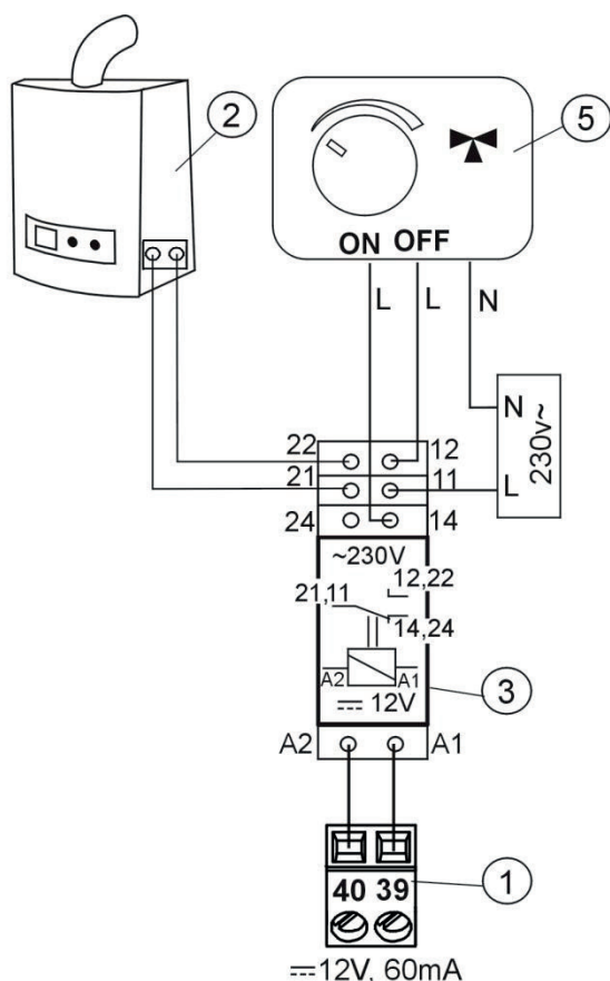
Rys. 20 Schemat elektryczny sterowania zaworem przełączającym kotła rezerwowego, gdzie: 1 – regulator, 2 – kocioł rezerwowy, 3 – przełącznik, 5 – siłownik zaworu przełączającego (z wyłącznikami krańcowymi), uwaga: zaciski 22,21,24 muszą być odseparowane galwanicznie od zacisków 12,11,14.
