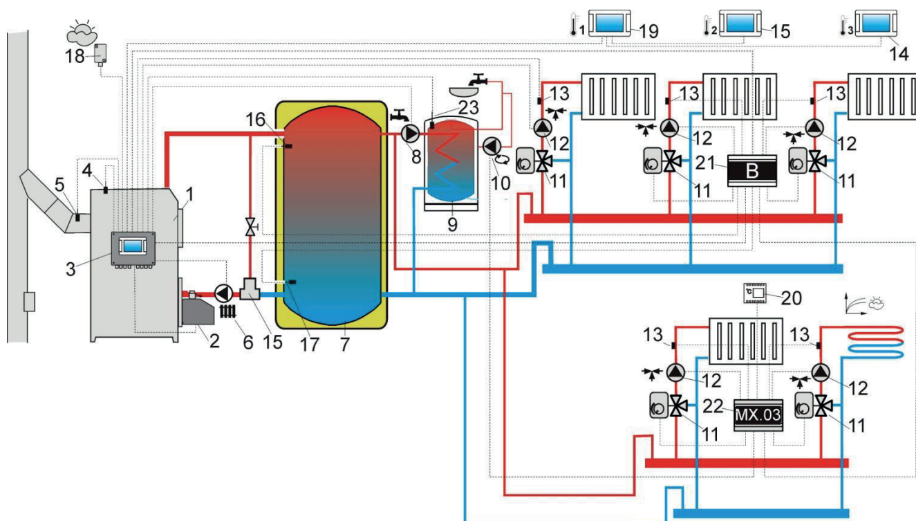
Rys. 12 Schemat z buforem cieplnym oraz z 5 mieszczowymi obiegami grzewczymi 3 , gdzie: 1 – kocioł, 2 – palnik, 3 – regulator, 4 – czujnik temperatury kotła CT4, 5 – czujnik temperatury spalin CT2S, 6 – pompa kotła, 7 – bufor cieplny, 8 – pompa ciepłej wody użytkowej, 9 – zasobnik ciepłej wody użytkowej, 10 – pompa cyrkulacyjna, 11 – zawór trójdrogowy z siłownikiem, 12 – pompa obiegu mieszacza, 13 – czujnik temperatury obiegu mieszacza CT4, 14 – panel pokojowy ecoSTER-TOUCH, 15 – panel pokojowy ecoSTER-TOUCH, 16 – czujnik górny temperatury bufora CT4, 17 – czujnik dolny temperatury bufora CT4, 18 – pogodowy czujnik temperatury CT4-P, 19 – panel pokojowy ecoSTER-TOUCH, 20 – standardowy termostat pokojowy (zwierno/rozwierny), 21 – dodatkowy moduł B, 22 – dodatkowy moduł MX.03, 23 – czujnik temperatury ciepłej wody użytkowej.
