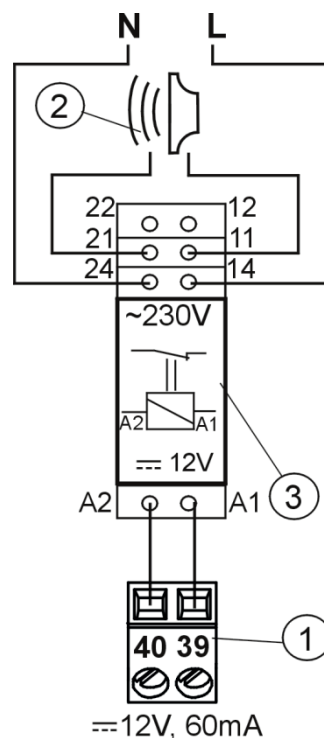
Rys. 21 Podłączenie zewnętrznego urządzenia alarmowego, gdzie: 1- regulator , 2 –zewnętrzne urządzenie alarmowe, 3 – przełącznik.
