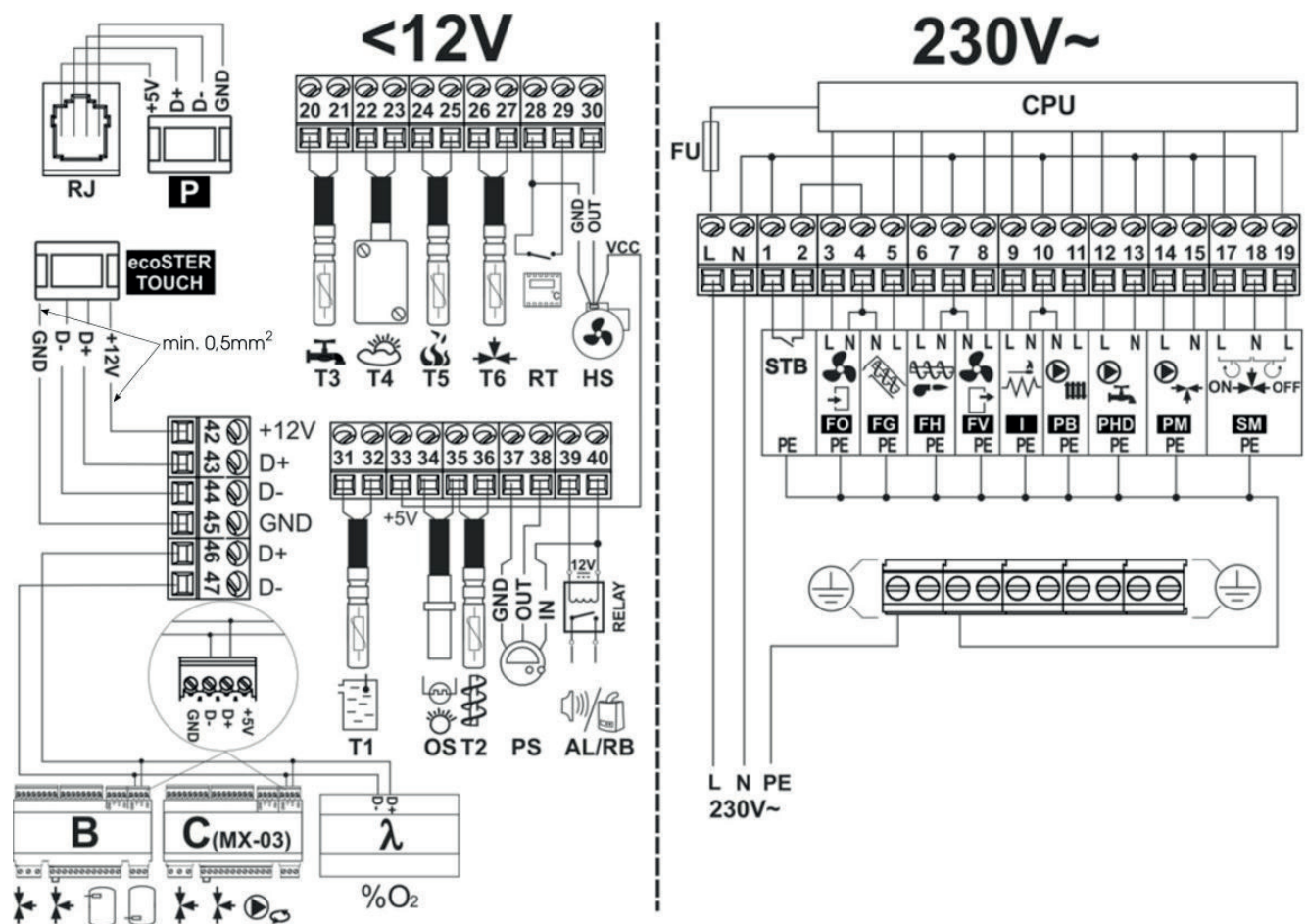
Rys. 15 Schemat połączeń elektrycznych regulatora , gdzie: T1 – czujnik temperatury kotła CT4, OS – czujnik optyczny płomienia, T2 – czujnik temperatury podajnika, PS – czujnik podciśnienia, AL/RB – wyjście napięciowe do sygnalizacji alarmów lub sterowania kotłem rezerwowym, T3 – czujnik temperatury ciepłej wody użytkowej CT4, T4 – pogodowy czujnik temperatury CT4-P, T5 – czujnik temperatury spalin CT2S, T6 – czujnik temperatury mieszacza CT4, RT – wejście termostatu pokojowego kotła, HS – czujnik obrotów wentylatora, P – panel sterujący, ecoSTER-TOUCH – panel pokojowy z funkcją termostatu pokojowego (zastępuje RT), D-D+ – złącze do dodatkowych modułów, B – moduł B powiększa o obsługę dodatkowych dwóch obiegów mieszaczy i obsługę bufora cieplnego, MX.03 – dodatkowy moduł powiększa o obsługę dodatkowych dwóch mieszaczy i pompę cyrkulacyjną, \lambda – moduł sondy Lambda, L N PE – zasilanie sieciowe 230V~, FU – bezpiecznik sieciowy, STB – wejście do ogranicznika temperatury bezpieczeństwa, FO – wentylator nadmuchiwy palnika, FG – podajnik główny, FH – podajnik palnika lub mechanizm obrotowego czyszczenia rusztu, FV – wentylator wyciągowy kotła, I – zapalarka, PB – pompa kotła lub bufora, PHD – pompa ciepłej wody użytkowej, PM – pompa mieszacza, SM – siłownik mieszacza, CPU – sterowanie.
