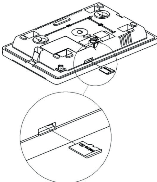
Rys. 22 Wkładanie karty pamięci microSD
