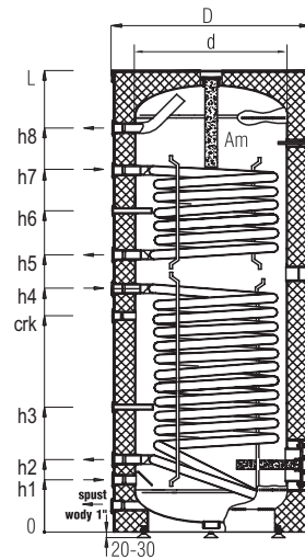
Wymiennik SGW(S)B 250, 400
