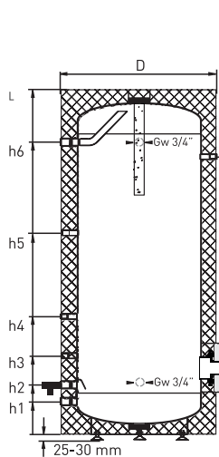
Zasobnik SG(S) 100-140
