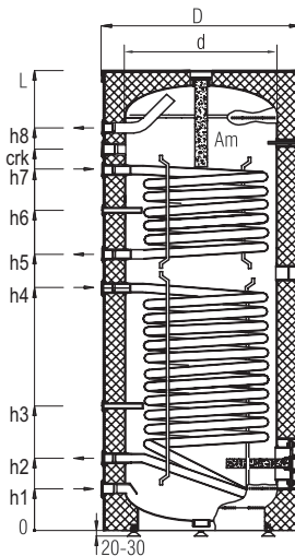
Wymiennik SGW(S)B 500, 1500
