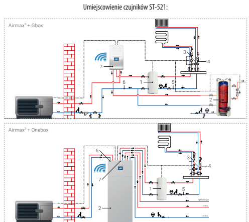
Rysunek 1: Poglądowe schematy instalacji z pompą ciepła Airmax² wraz z oznaczeniami czujników. W opisie parametrów ekranu szczegółowego zawarto odpowiednie numery czujników.
