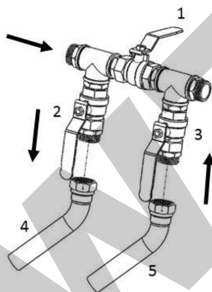
Rysunek 4 Zestaw napełniający, lokalizacja w instalacji dolnego źródła
